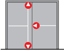
Çift kanat - 3 noktadan kilitleme
